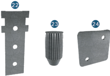
Kasnak Kayış Sıkıştırma T Sac Product Code: GYT-22 Quantity: 4 piece Kayış Bağlantı Pimi Product Code: GYT-23 Quantity: 2 piece Kayış Alt Sıkıştırma Product Code: GYT-24 Quantity: 4 piece
