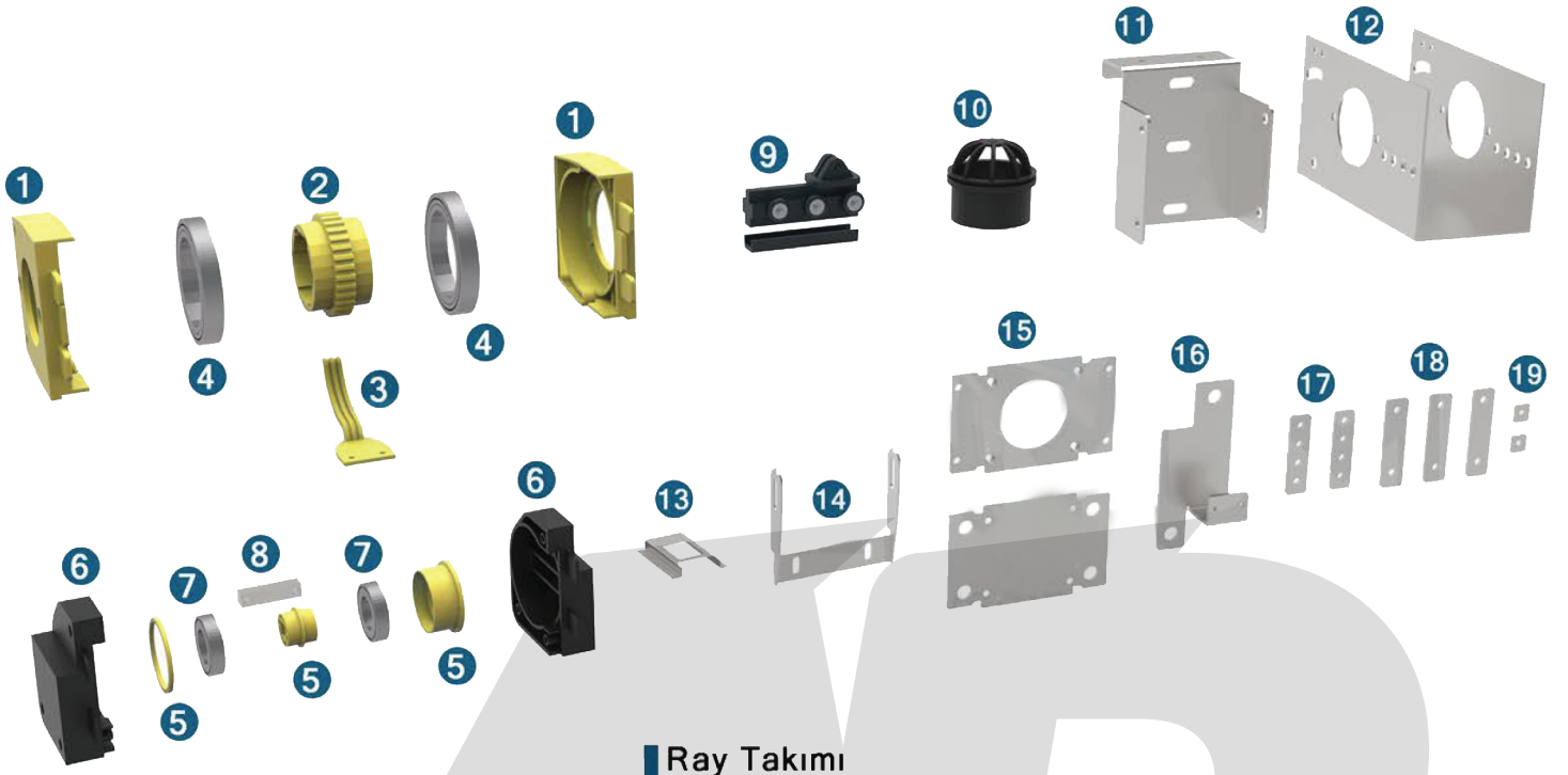
Ray Takımı Rail Set Product Code: Roll-01
