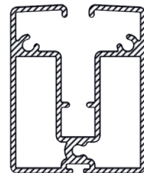
Saçak Profili Fringe Profile
